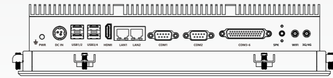
选项3: 2网口+4USB+6COM+1功放+WIFI
