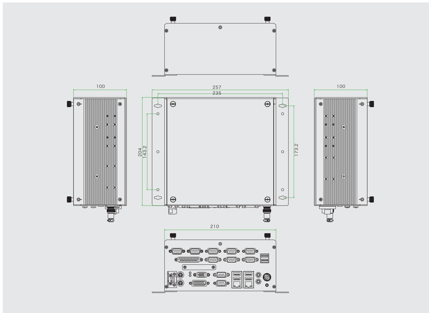
尺寸图:
